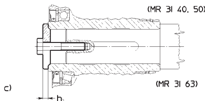
Fissaggio assiale Axial fastening
