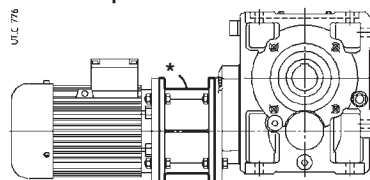
MLS / MLA montaggio tra riduttore e motore o motorizzatore mounted between gear reducer and motor or motor-variator
