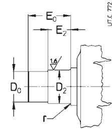
e) Perno macchina «corto» e) «Short» shaft end of driven machine
