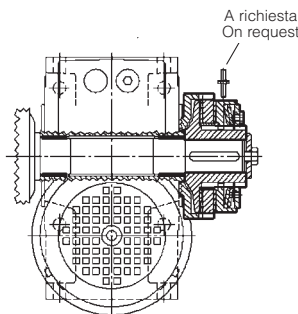
Montaggio limitatore esterno External limiter mounting
