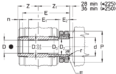
c) Albero lento cavo differenziato con unità di bloccaggio e perno macchina «lungo» c) Stepped hollow low speed shaft with locking assembly and «long» machine shaft end
