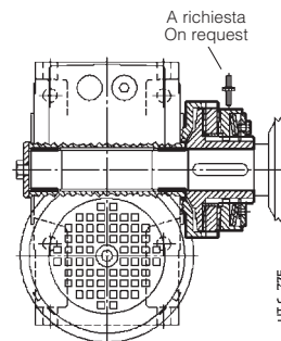
Montaggio limitatore intermedio Intermediate limiter mounting
