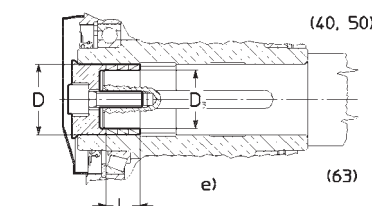
Callettamento con linguetta e anelli di bloccaggio e), con linguetta e bussola di bloccaggio f). Fitting with key and locking rings e), with key and locking bush f).
